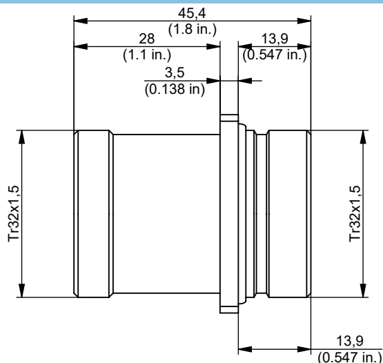
Einbaumaße / Mounting dimensions
