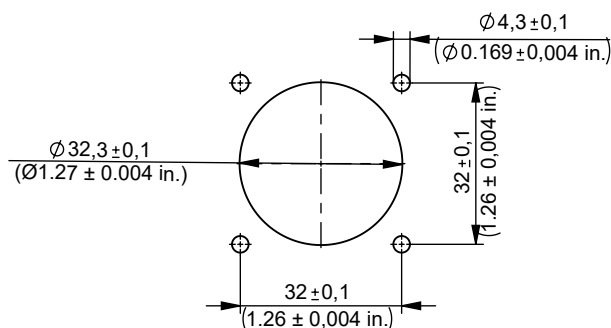
Einbaumaße / Mounting dimensions
