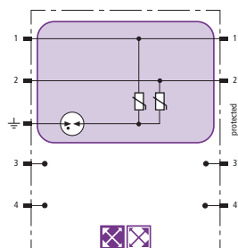
Prinzipschaltbild
